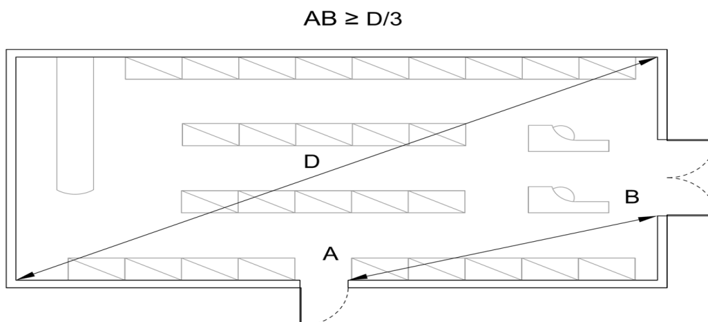
Σχήμα 1 Διάταξη τελικών εξόδων
